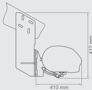
Stiprina pie spārēm Roof rafter installation Монтаж к кровли
