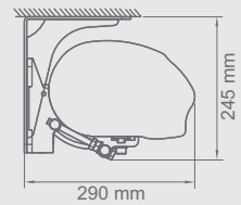
Stiprina pie griestiem Ceiling installation Потолочная установка
